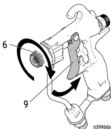
FIG. 52: Presionar el gatillo mientras enrosca el cartucho
