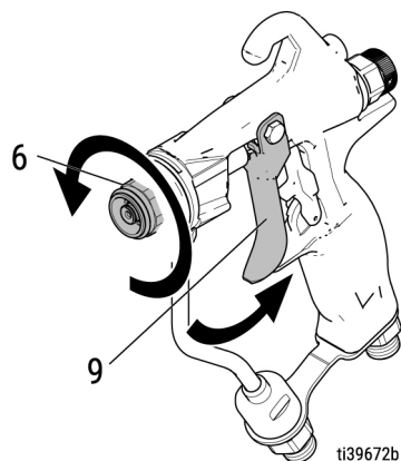
FIG. 50: Quitar el cartucho de fluido
